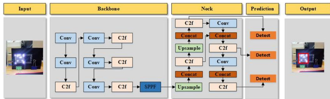
Gambar 2.7 Arsitektur YOLOv8
