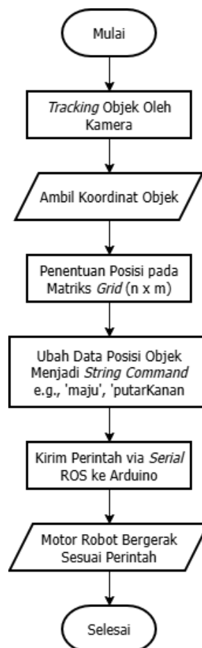
Gambar 3.5 Flowchart Kerja Algoritma Lokalisasi Grid
